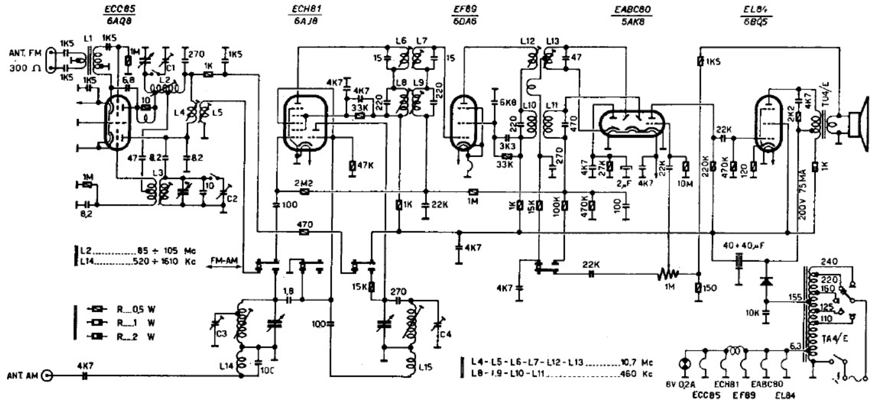
SCHEMA ELETTRICO DEL RADIORICEVITORE G.B.C. FM/1A 1° DANDY
